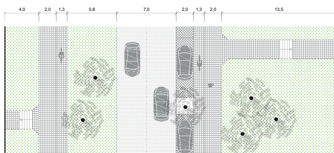
SKUTECKÉHO - NÁVRH
